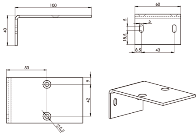
Guide rail (7-303770-0000)
